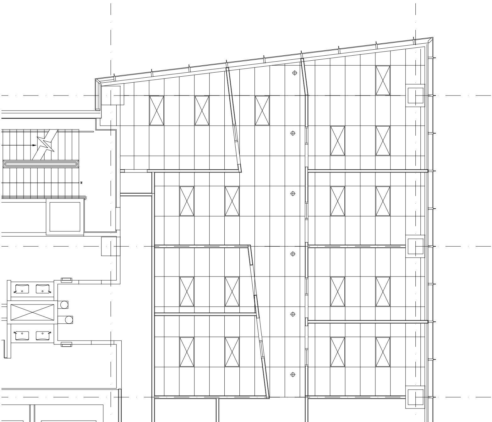
REFLECTED CEILING SCALE: 1/8" = 1'-0"
